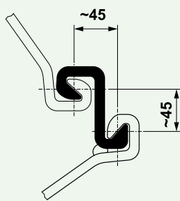
C 14 Ciężar ~ 14,4 kg/m
