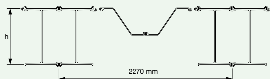
Ścianka kombinowana HZ.....-24 / AZ 18
