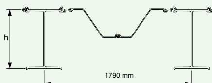
Ścianka kombinowana HZ.....-12 / AZ 18
