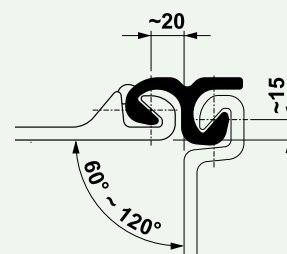
DELTA 13 Ciężar ~ 13,1 kg/m
