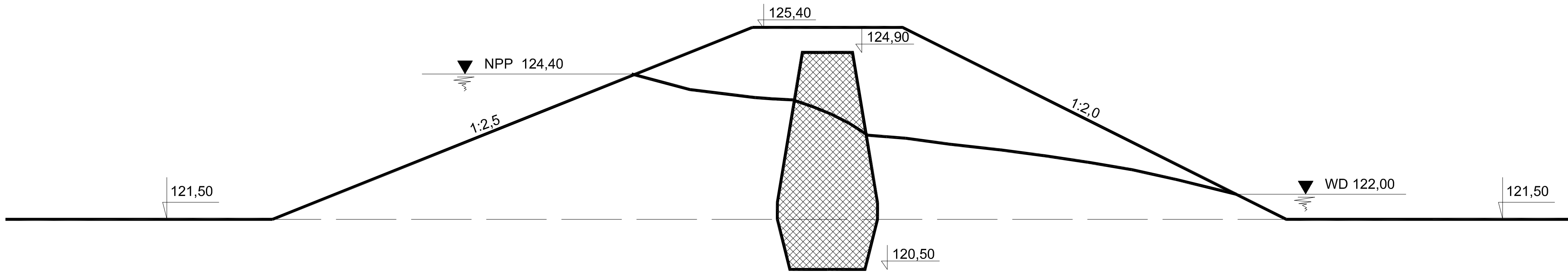
Przekrój B - B
