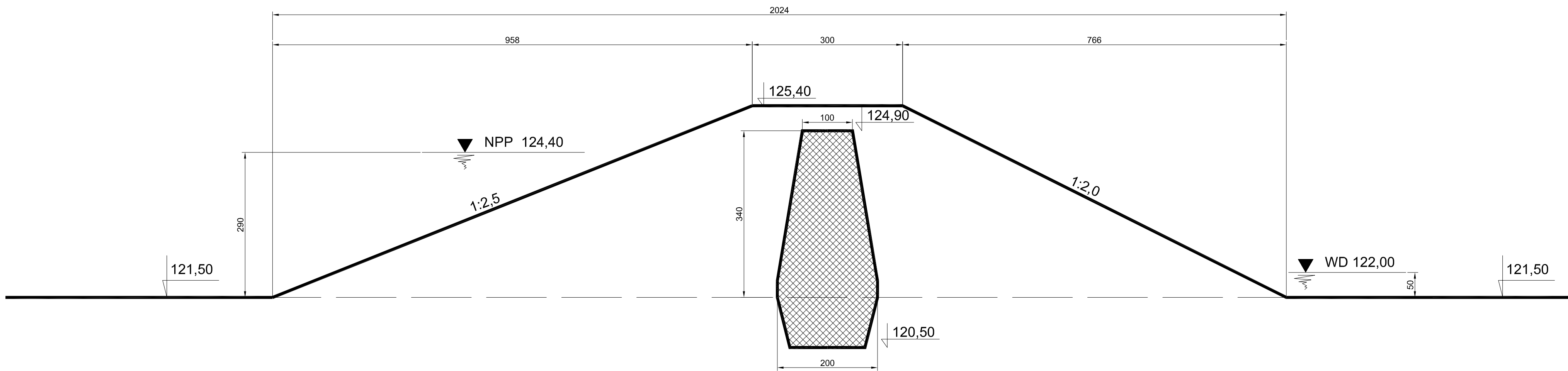
Przekrój B - B
